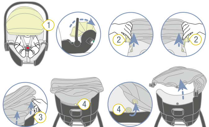
1 Sonnenverdeck 2 Steckzungen 3 Babyschalen-Rand 4 Druckknopf
